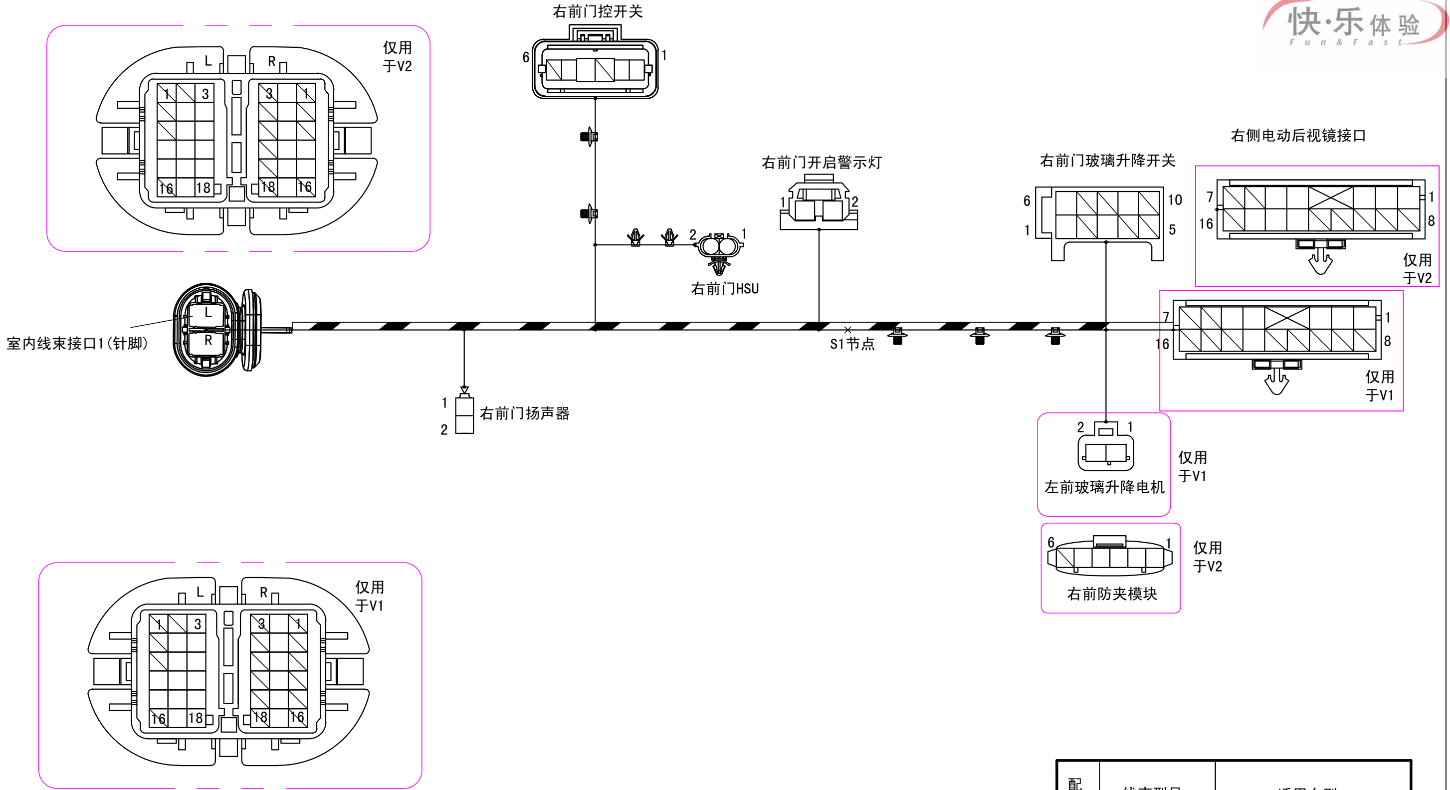
2. 26、右前门线束插件端子图
